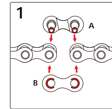
A. Sigma Pro link B. Sigma Pro top plate
